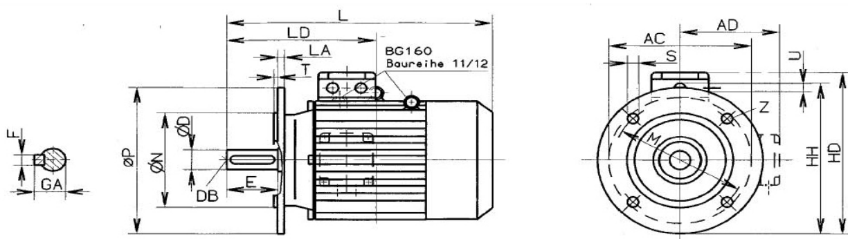
2 polni motorji (2800 obr.) IM B5 (prirobnica)
